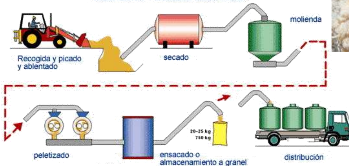
ESQUEMA DE PRODUCCIÓN DEL PELLET
